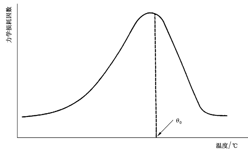
图5 典型的力学损耗因数曲线
